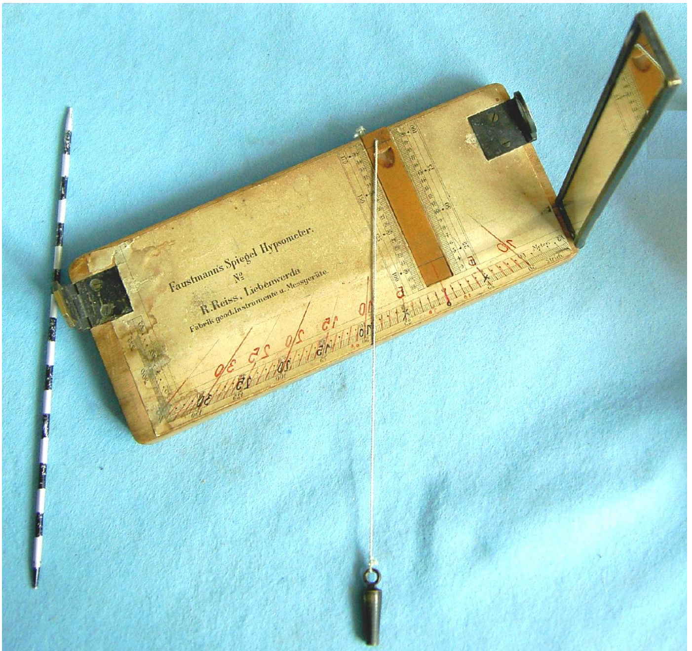
Sammlung Wolfgang Rucker: Faustmann Spiegel-Hypsometer (ab 1854) zur Baumhöhenmessung mit Senklot
